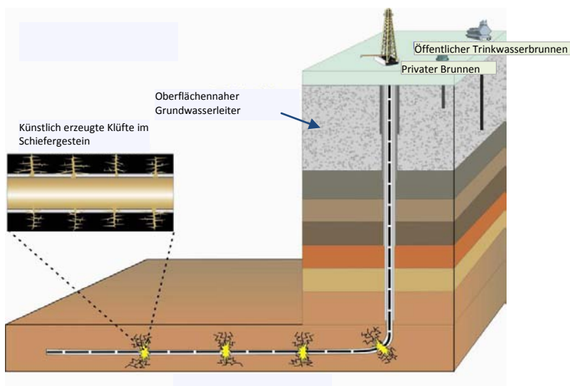
Abbildung 2 Schematische Darstellung einer horizontal abgelenkten Bohrung in einen Schiefergashorizont (US EPA Hydraulic Fracturing Research Study, 2010)
